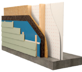
Murs Extérieurs Isolation des murs extérieurs avec structure de bois
