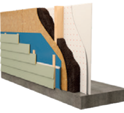
Murs Extérieurs Isolation intérieure des murs extérieurs
