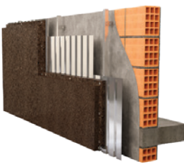
Murs Extérieurs Revêtement extérieur visible avec système de fixation mécanique
