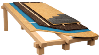
Toitures Toiture inclinée avec isolation audessus des chevrons
